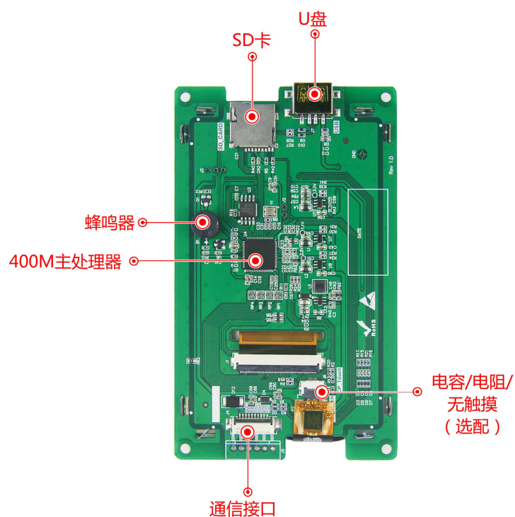
图 1-4 硬件配置图
