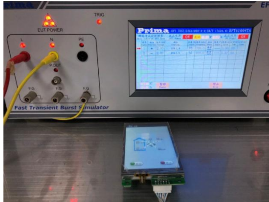
图 4-3 EFT 测试图
