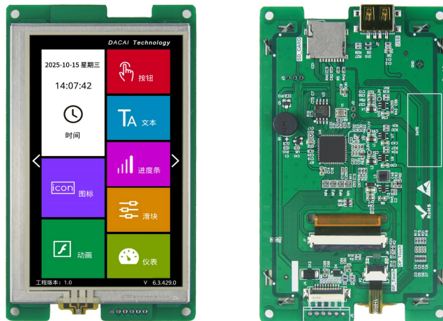
图 1-2 4.3 寸电阻触摸参考图
