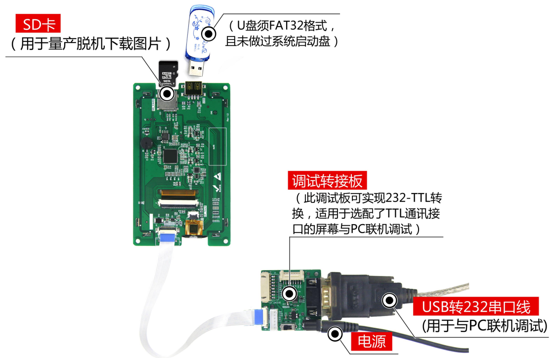
图 1-5 调试工具图
