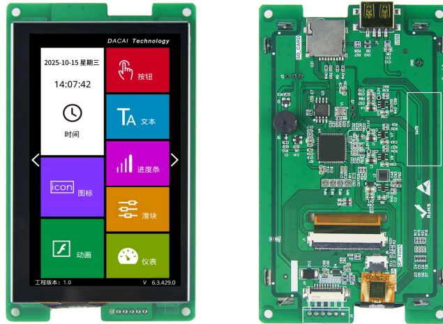
图 1-1 4.3 寸电容触摸参考图
