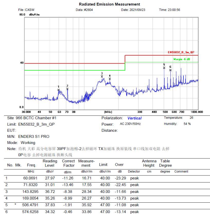
图 4-6 RE 测试垂直方向
